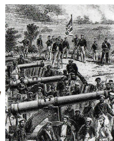
図5 砲台占領
